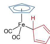
dicarbonyl(η 5 -cyclopentadiëno)(cyclopenta-2,4-dien-1-ido-κC 1 )ijzer of dicarbonyl(η 5 -cyclopentadiënyl)(cyclopenta-2,4-dien-1-yl-κC 1 )ijzer
